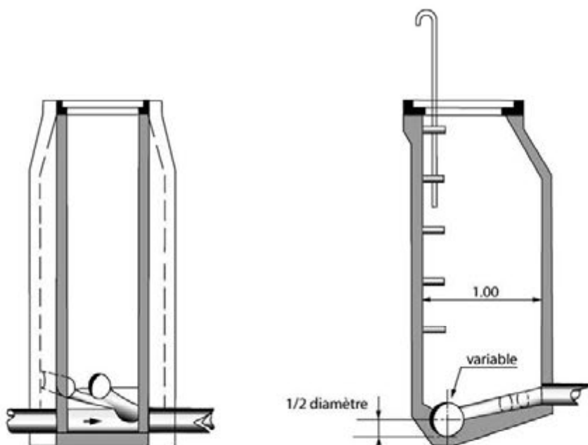
COUPE A-A
