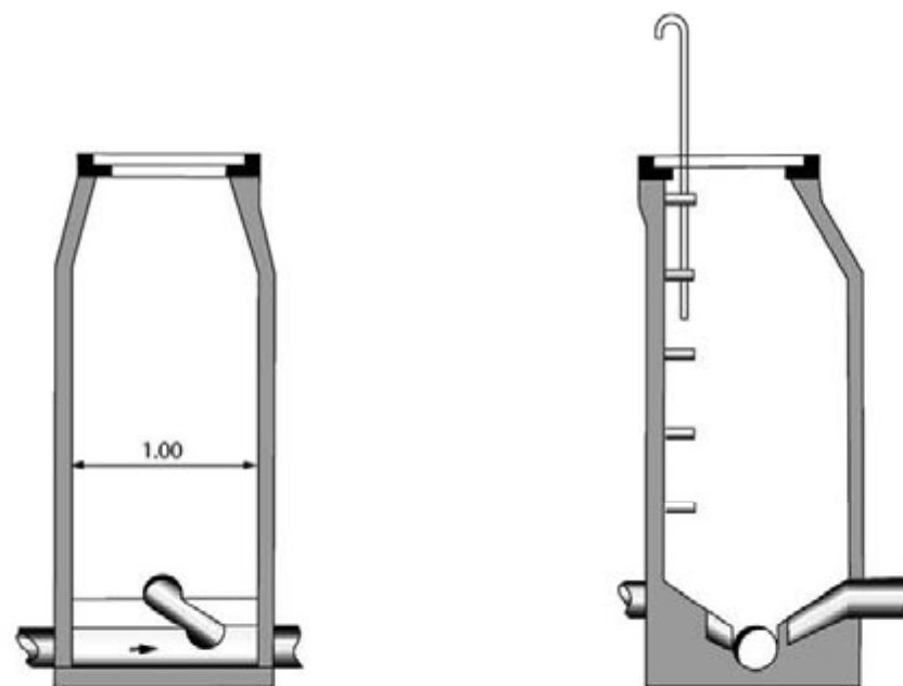
COUPE B-B
