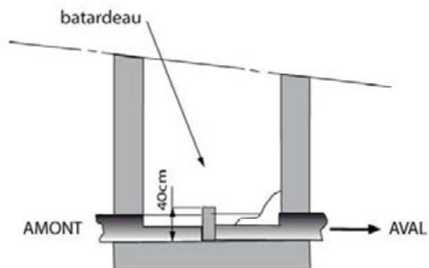
COUPE A-A
