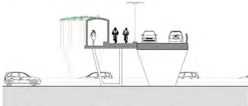
Pont Rue du Stade, coupe du projet
